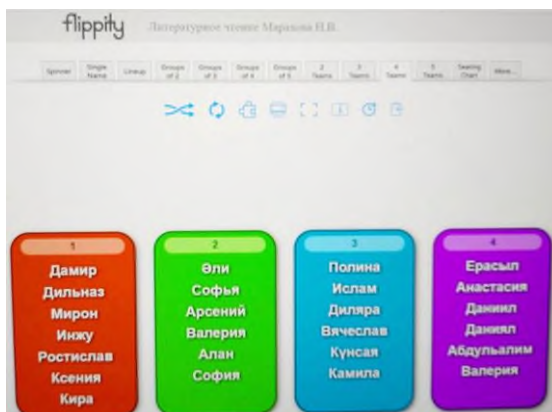
Рисунок 3.Рандомизатор Flippity.
